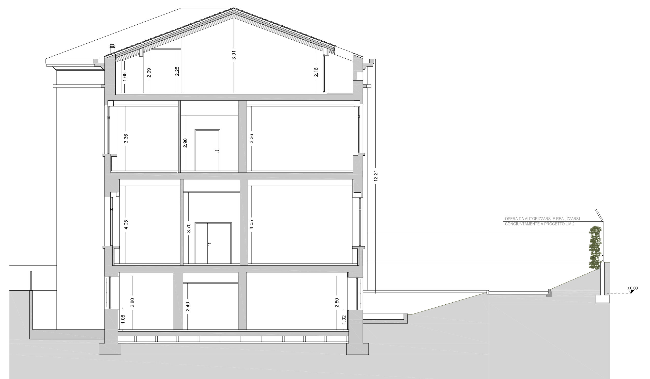
SEZIONE BB
