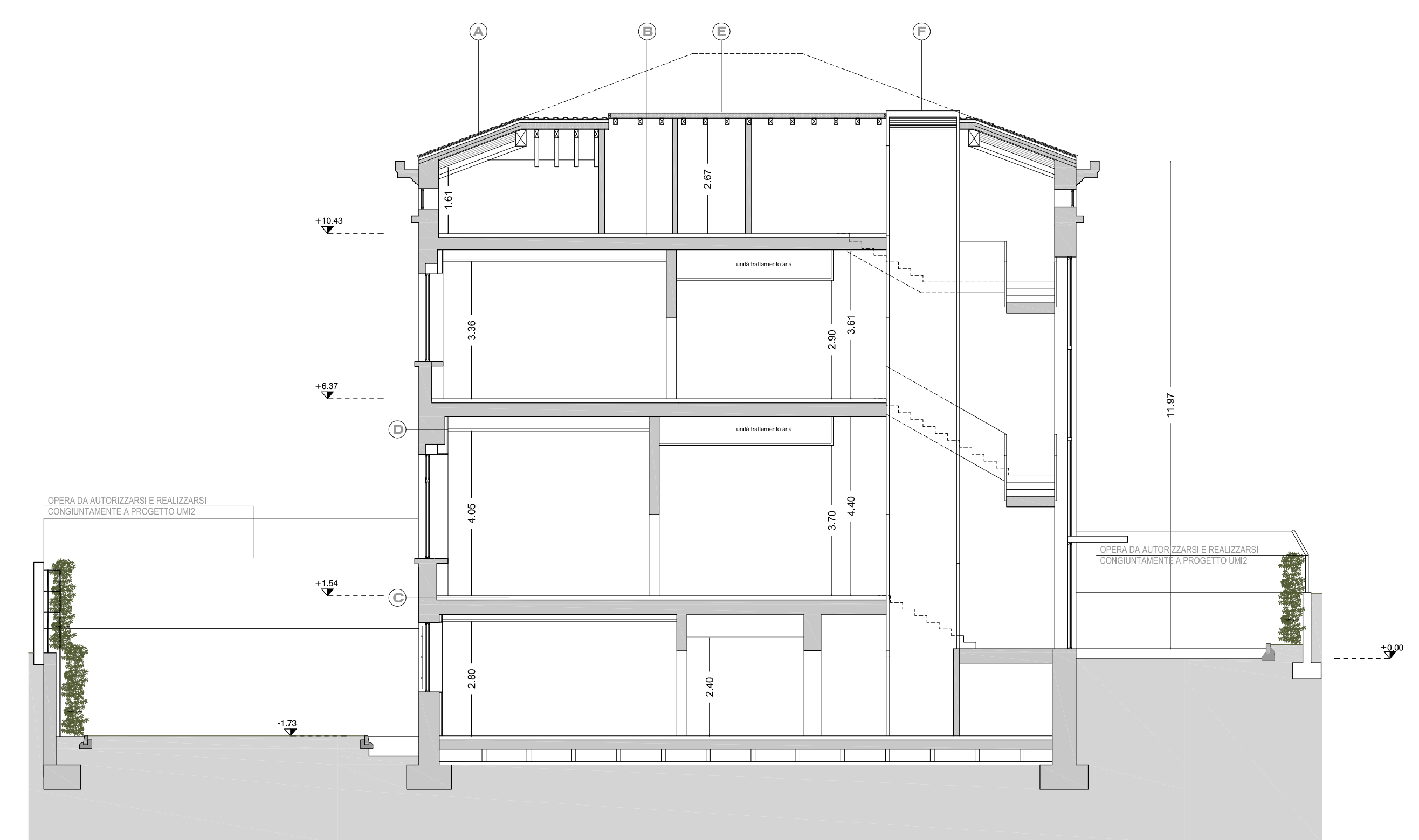
SEZIONE CC
