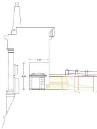
SEZIONE A-A COMPARATIVA
