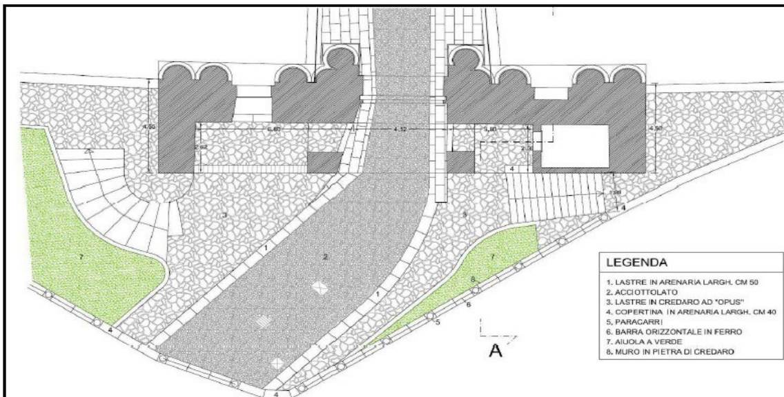
PLANIMETRIA STATO DI FATTO
